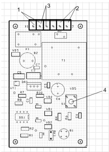
Рис. 5 - Схема соединения винтового клеммника на плате сигнализаторов СКЗП-МЕ-1 с внешними устройствами.
