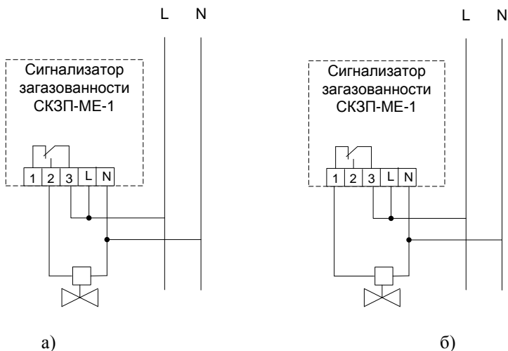
Рис. 3 - Схема соединения сигнализаторов СКЗП-МЕ-1 с внешней цепью: а) подключение газового клапан 220В типа НО; б) подключение газового клапан 220В типа НЗ.
