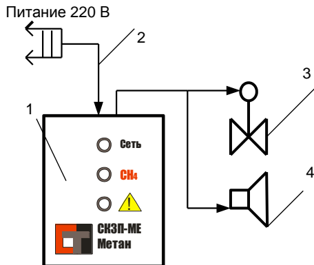
Рис. 1 - Сигнализатор загазованности СКЗП-МЕ: 1 - блок датчика; 2 - кабель питания с вилкой; 3 - клапан электромагнитный газовый; 4 - внешнее исполнительное устройство.
