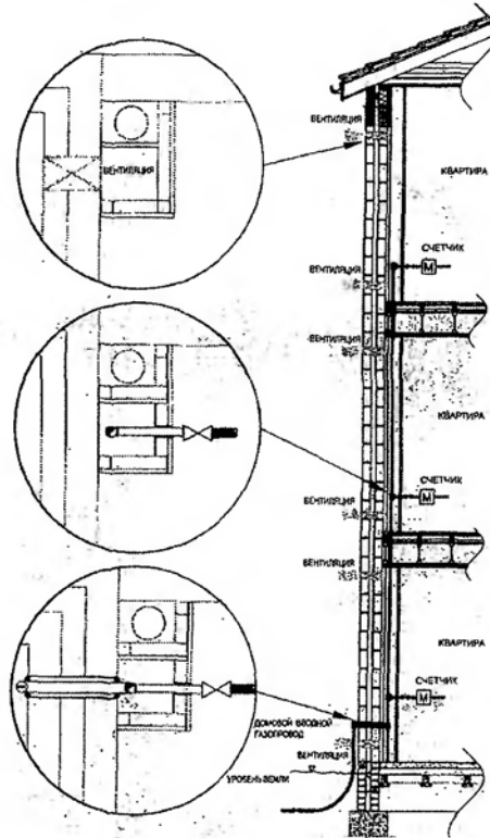
Рисунок Г.1 — Газопровод в вентилируемой штрабе
